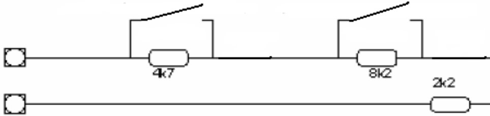
3 lü direnç bağlantısı
